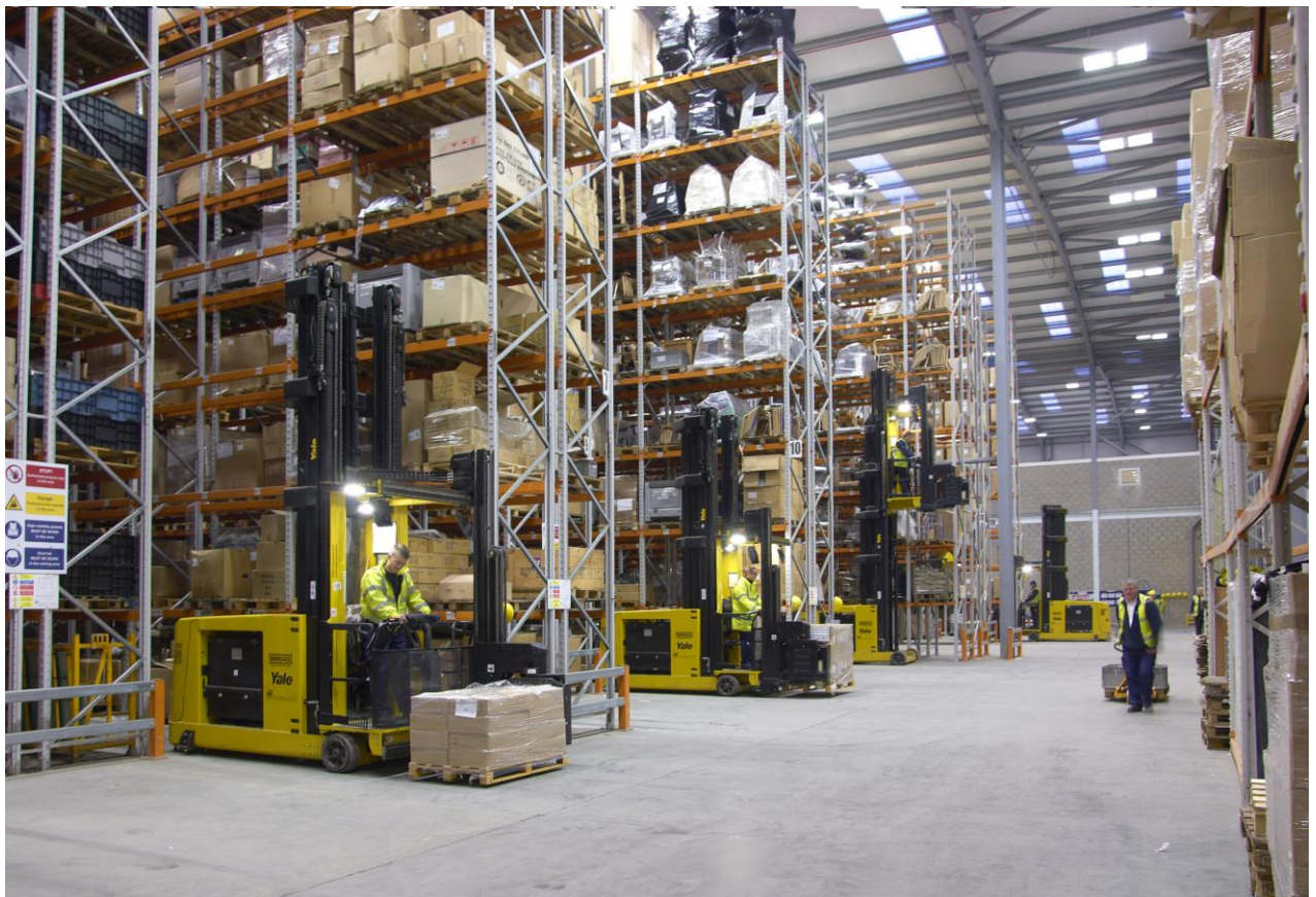
FOTO YALE VNA trucks, fabricate in Masate, Italia, livrate la Philips Orastie Inaltimi de ridicare de pana la 17 m
